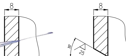
Detail I (详图 I)
